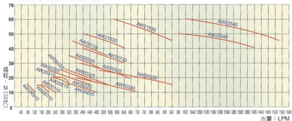
AW型2P(2極)三相性能表[60Hz(3500R.P.M.)]
