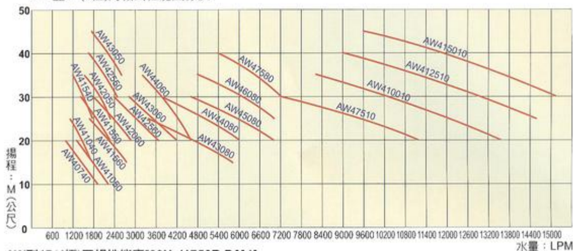
AW型4P(4極)三相性能表[60Hz(1750R.P.M.)]
