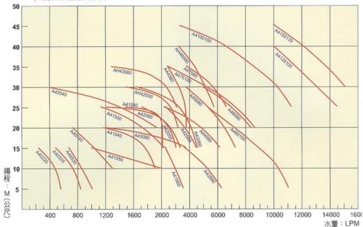
4P(4極)三相性能表[60Hz(1750R.P.M.)]
