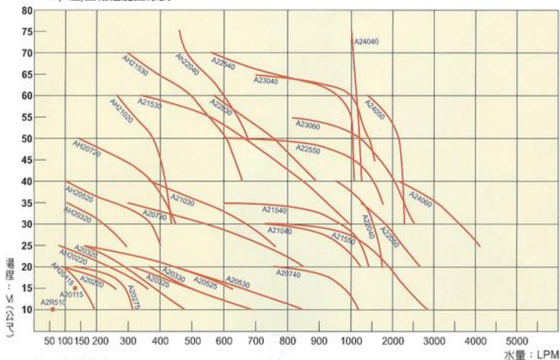
2P(2極)三相性能表[60Hz(3500R.P.M.)]
