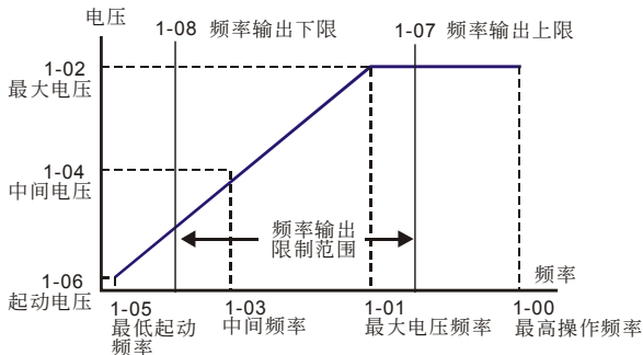
V/F曲线
