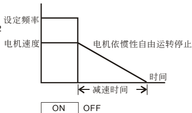
图二：自由运转
