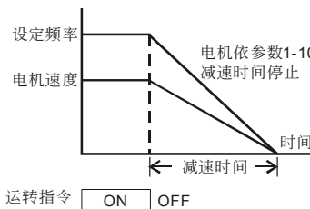
图一：减速刹车
