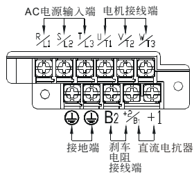
电源端子
