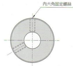
圖一 固定螺絲式 Set screw type
