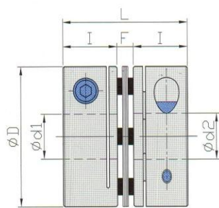
外徑 \phi 27 \sim \phi 34
