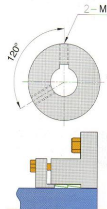
圖二 夾緊式 clamp type
