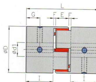
外徑 \phi 40 \sim \phi 65
