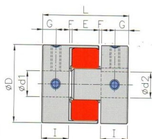
外徑 \phi 20 \sim \phi 30
