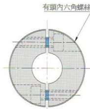
圖二 夾緊式 clamp type
