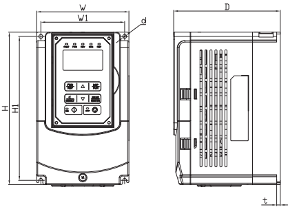
外型圖 A
