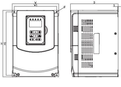
外型圖 B
