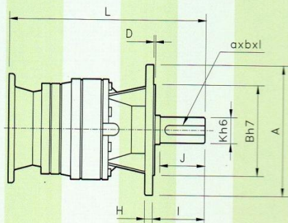
尺寸規格表 DIM.TABLE(mm)
