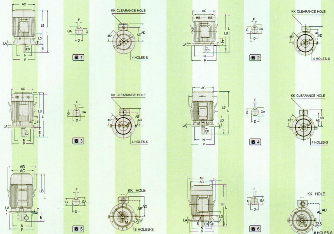
外形尺寸圖 (僅供參考)
