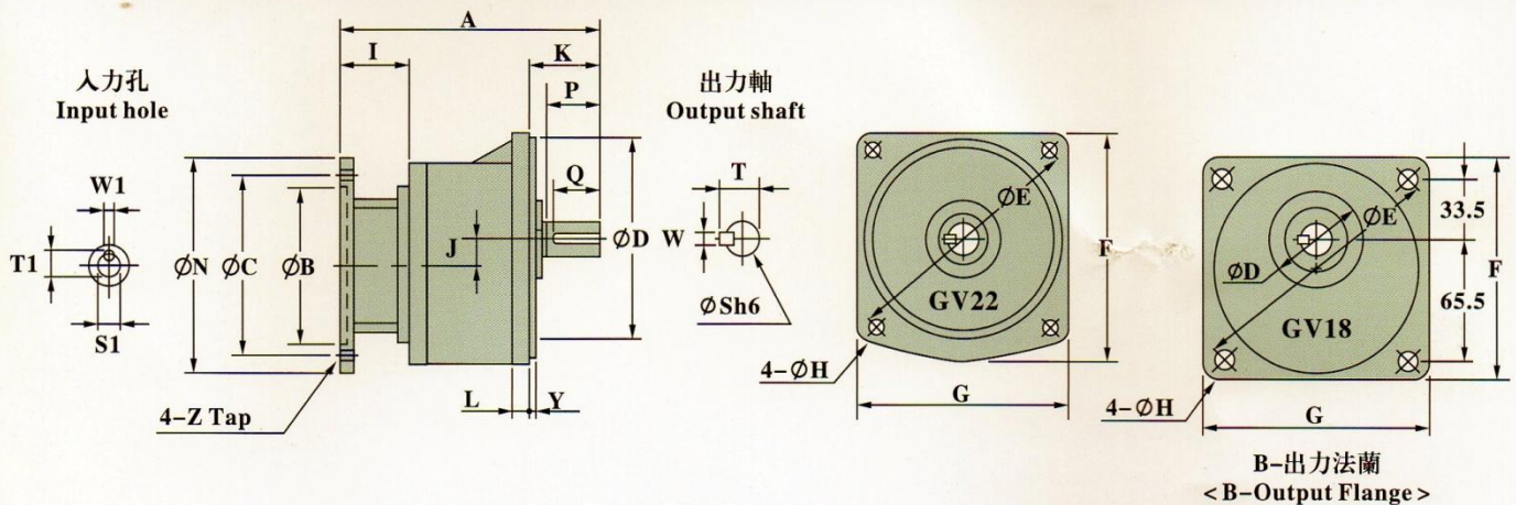
尺寸表(m/m)
