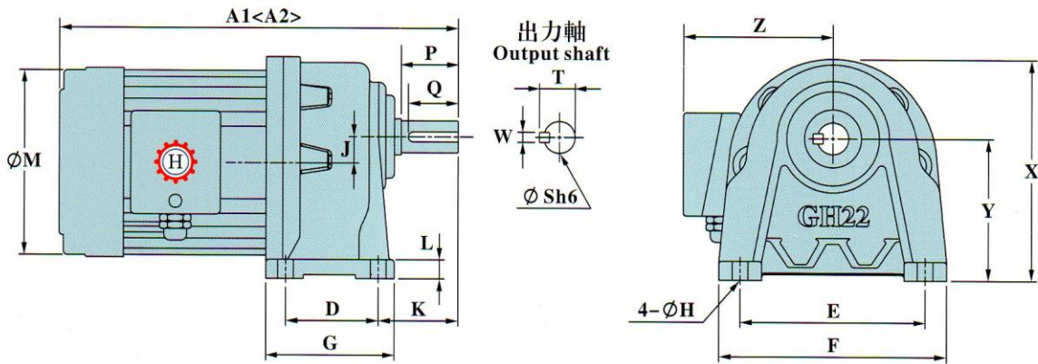
尺寸表(m/m)
