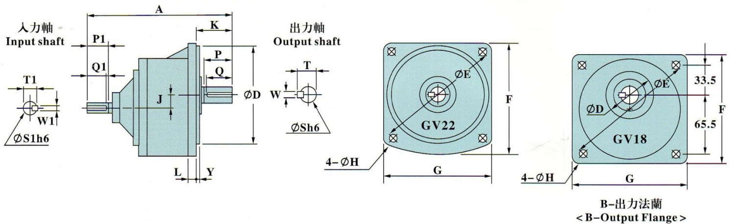
尺寸表(m/m)
